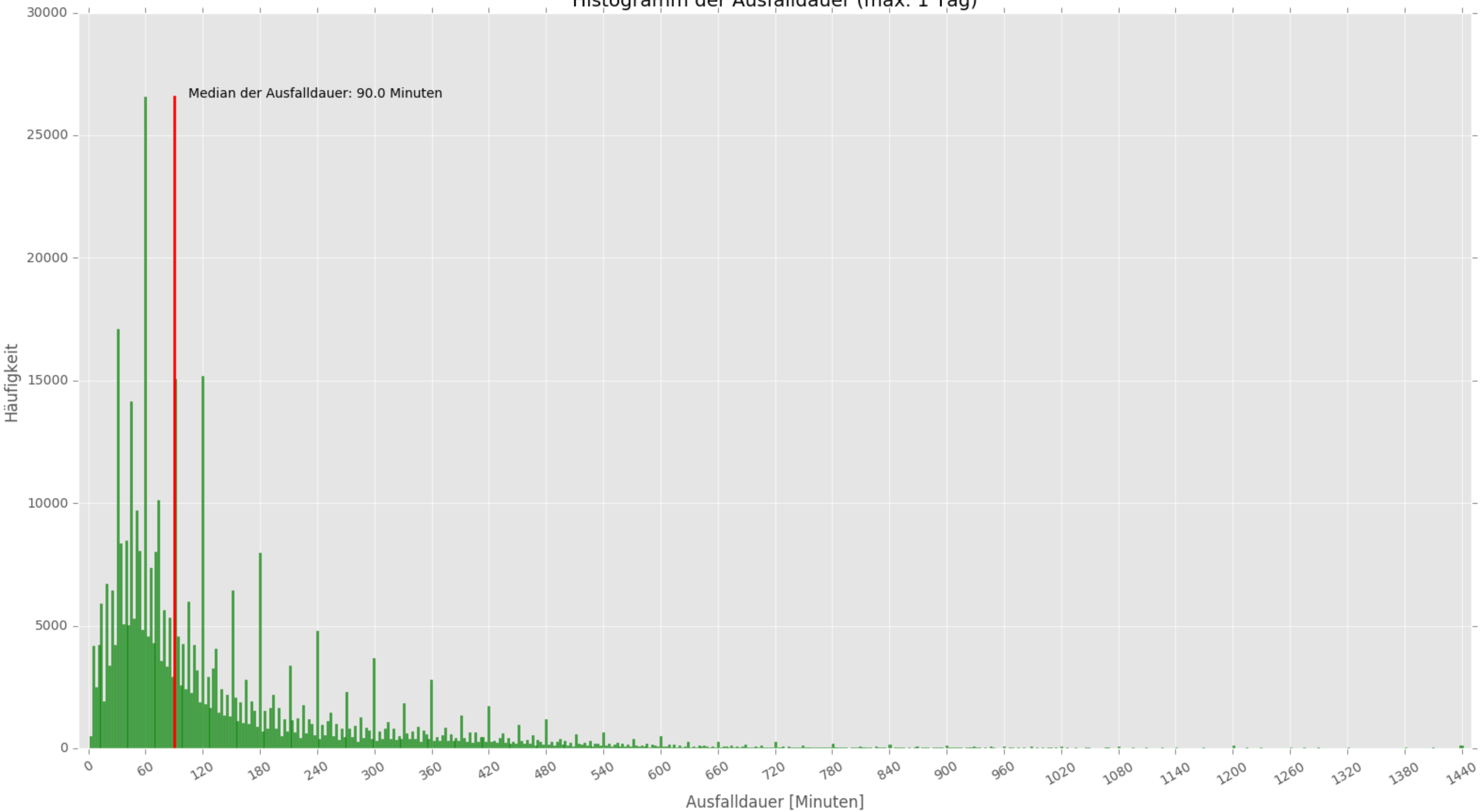
Histogramm der Ausfalldauer (max. 1 Tag)
