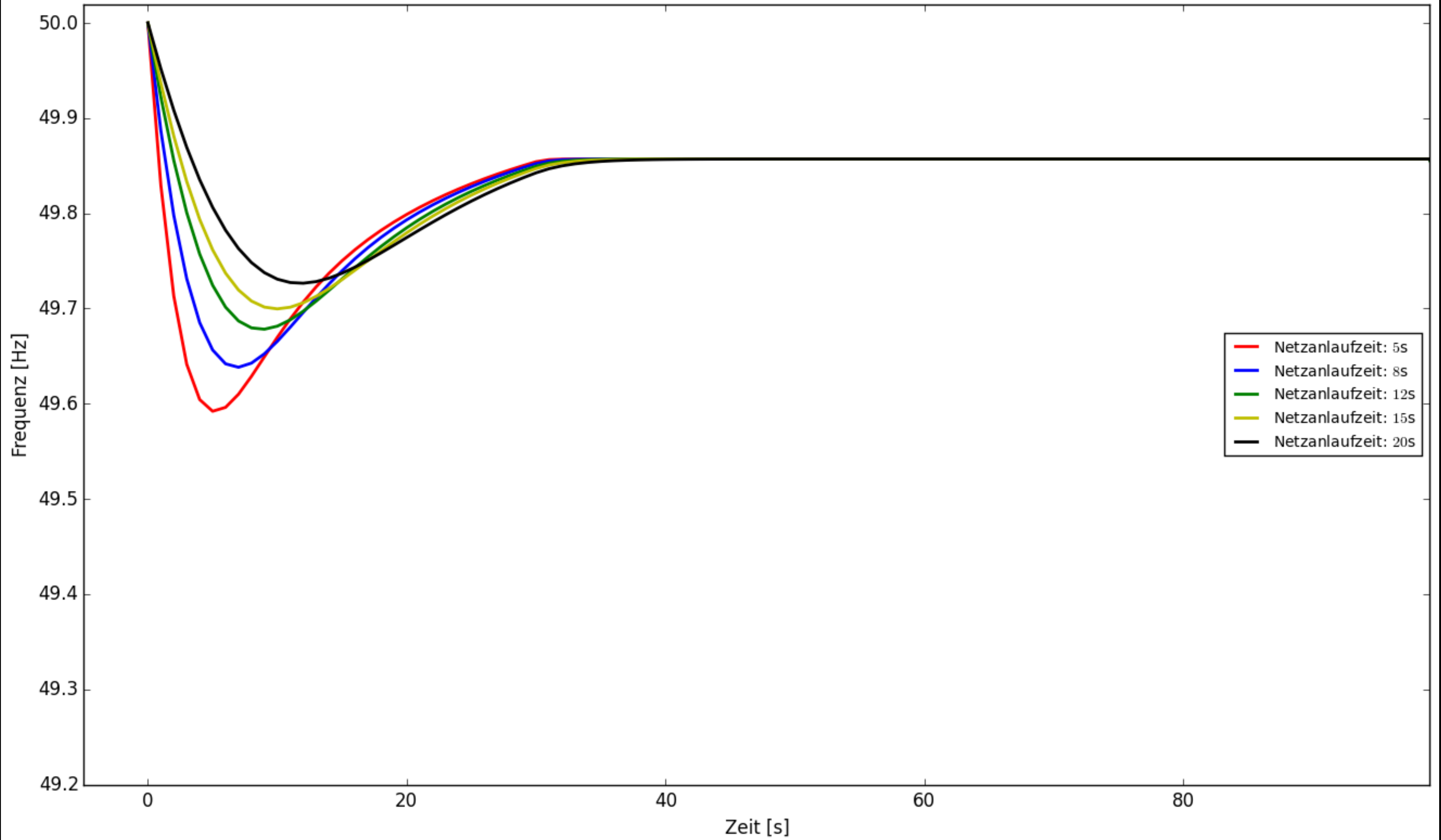
Netzlast 150.0 GW: Event von -3.00 GW
