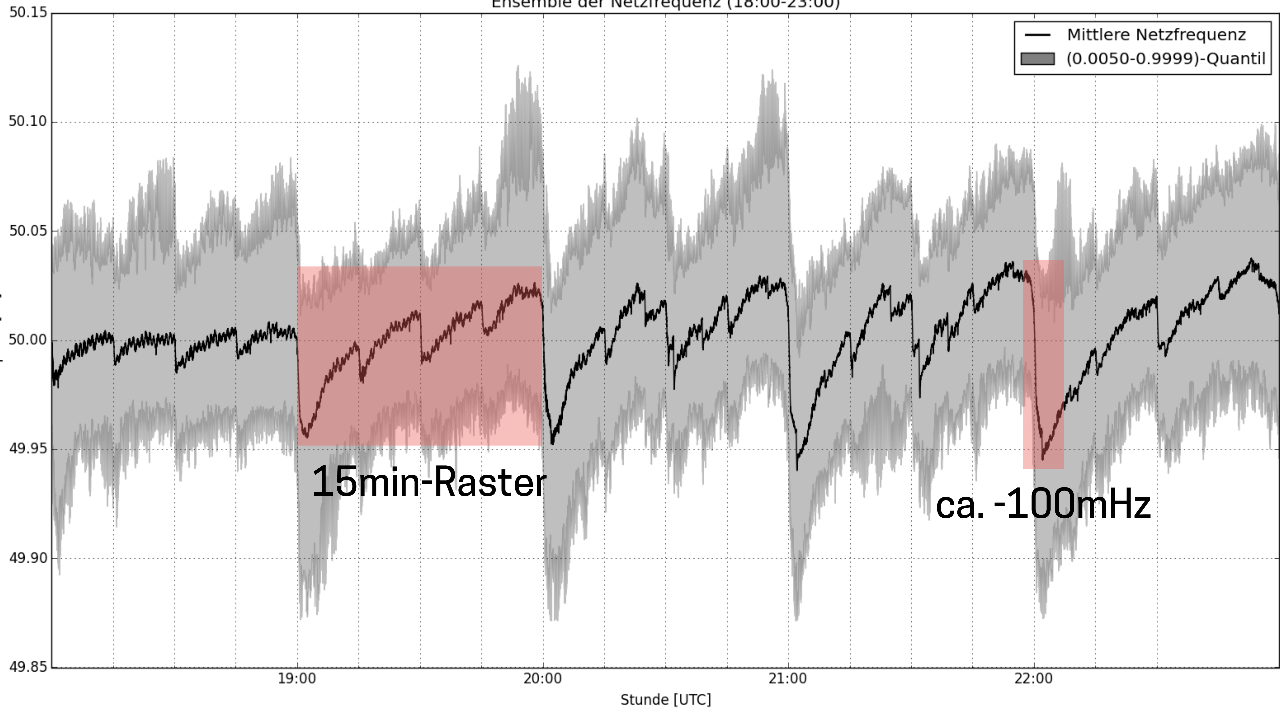
Ensemble der Netzfrequenz (18:00-23:00)
