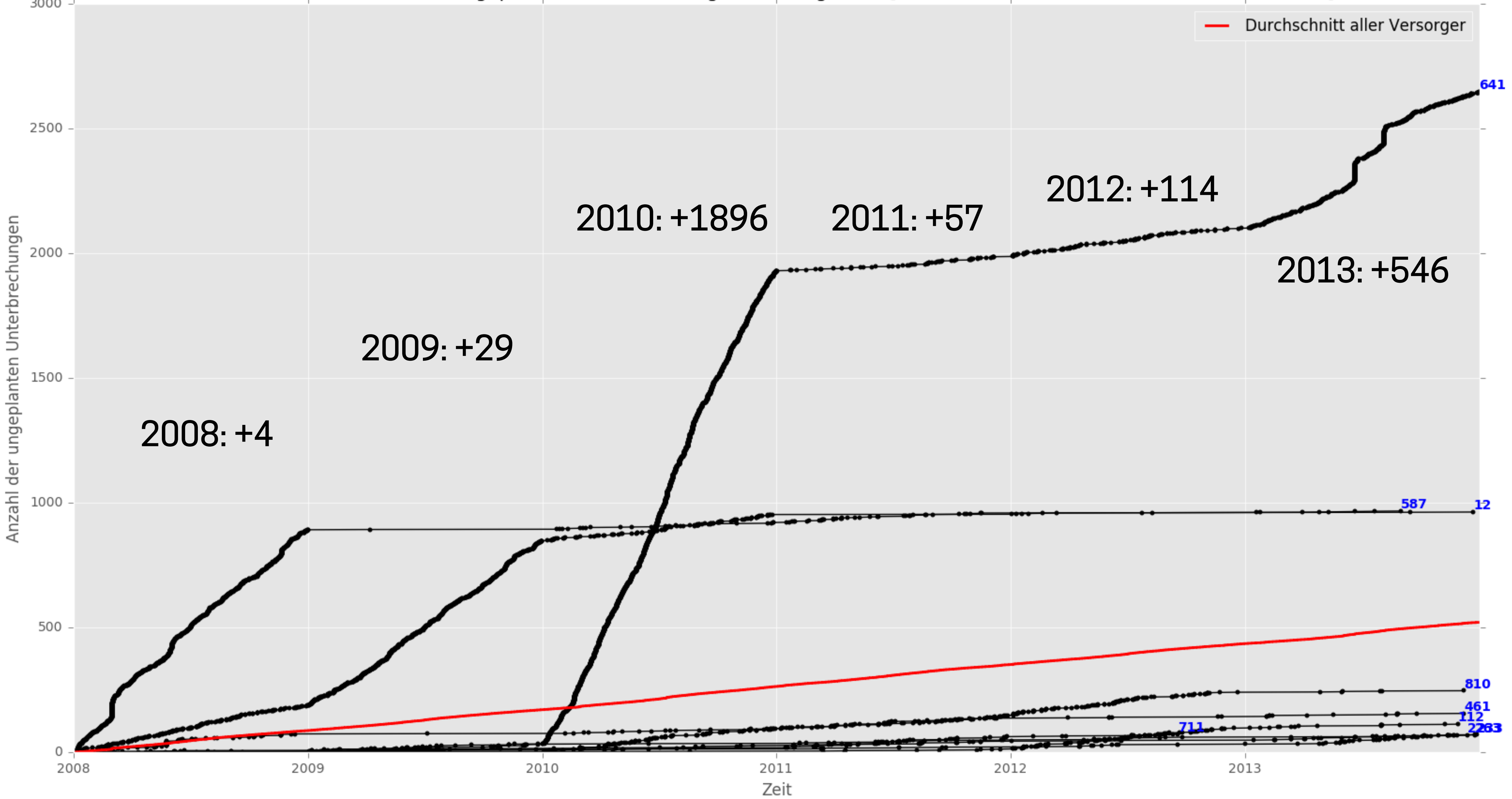
Kummulierte Anzahl der ungeplanten Unterbrechungen, Versorger-ID=[233, 810, 12, 641, 587, 711, 263, 2, 461, 112]
