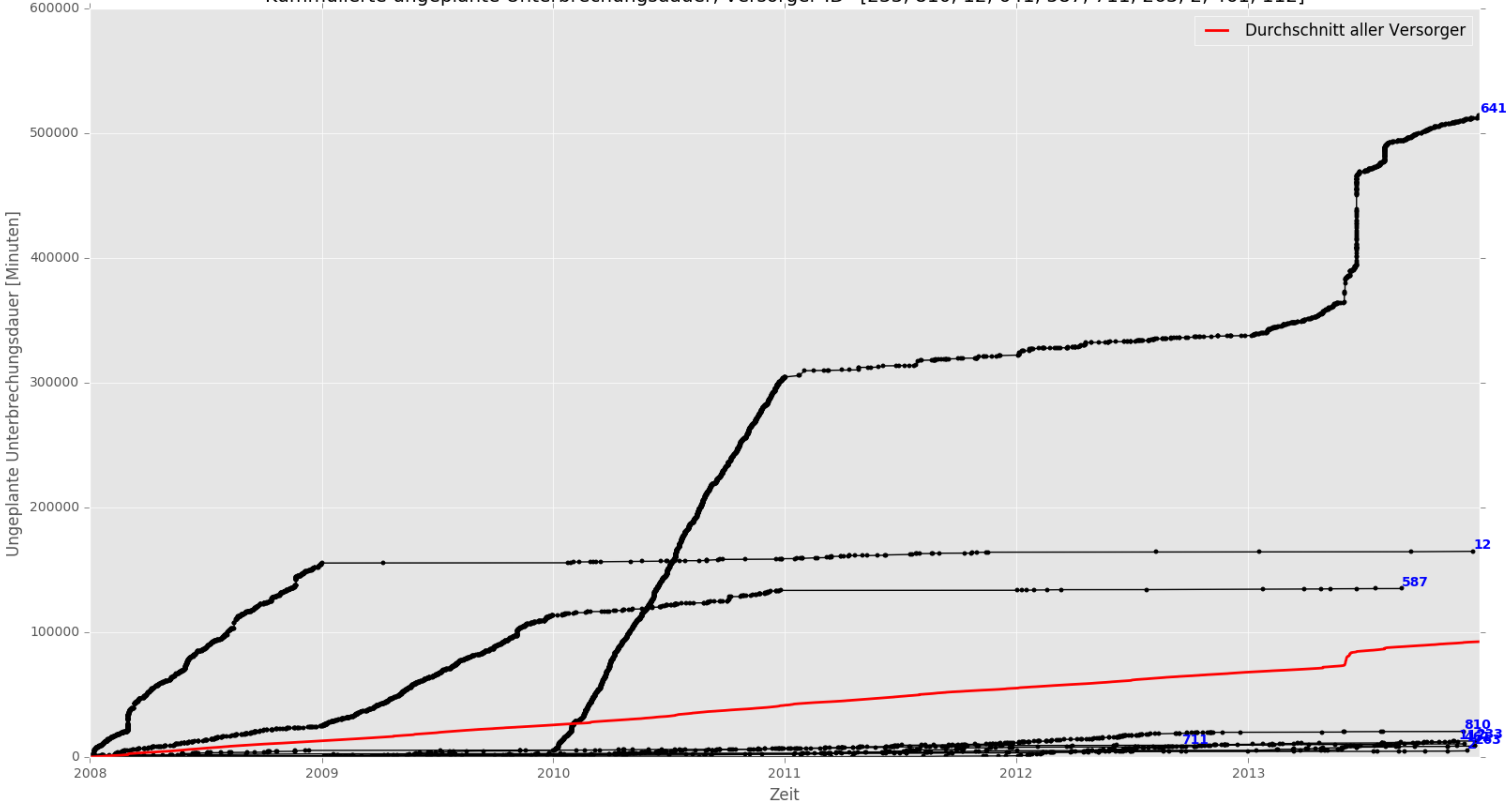
Kummulierte ungeplante Unterbrechungsdauer, Versorger-ID=[233, 810, 12, 641, 587, 711, 263, 2, 461, 112]
