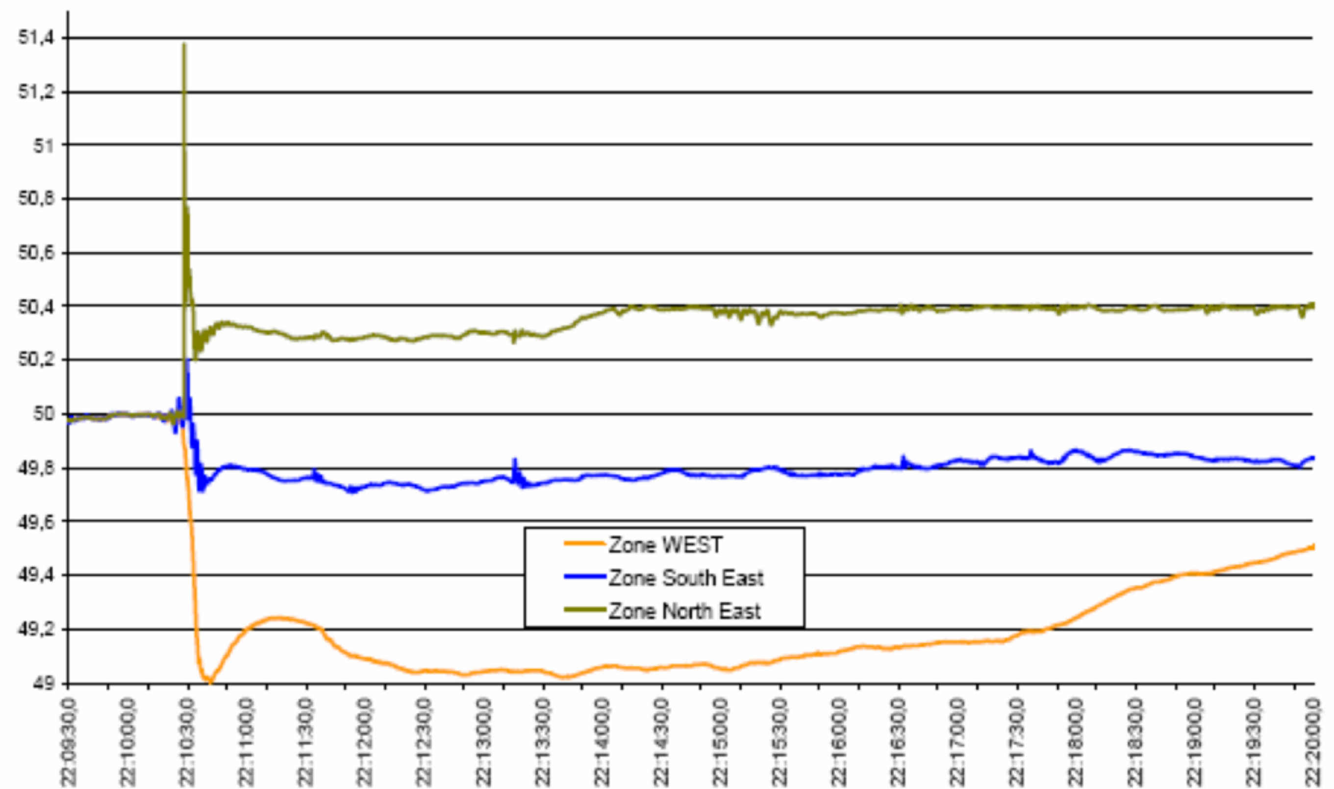
Abbildung 4: Aufzeichnungen der Frequenzen ab der Teilung des UCTE-Verbundnetzes
