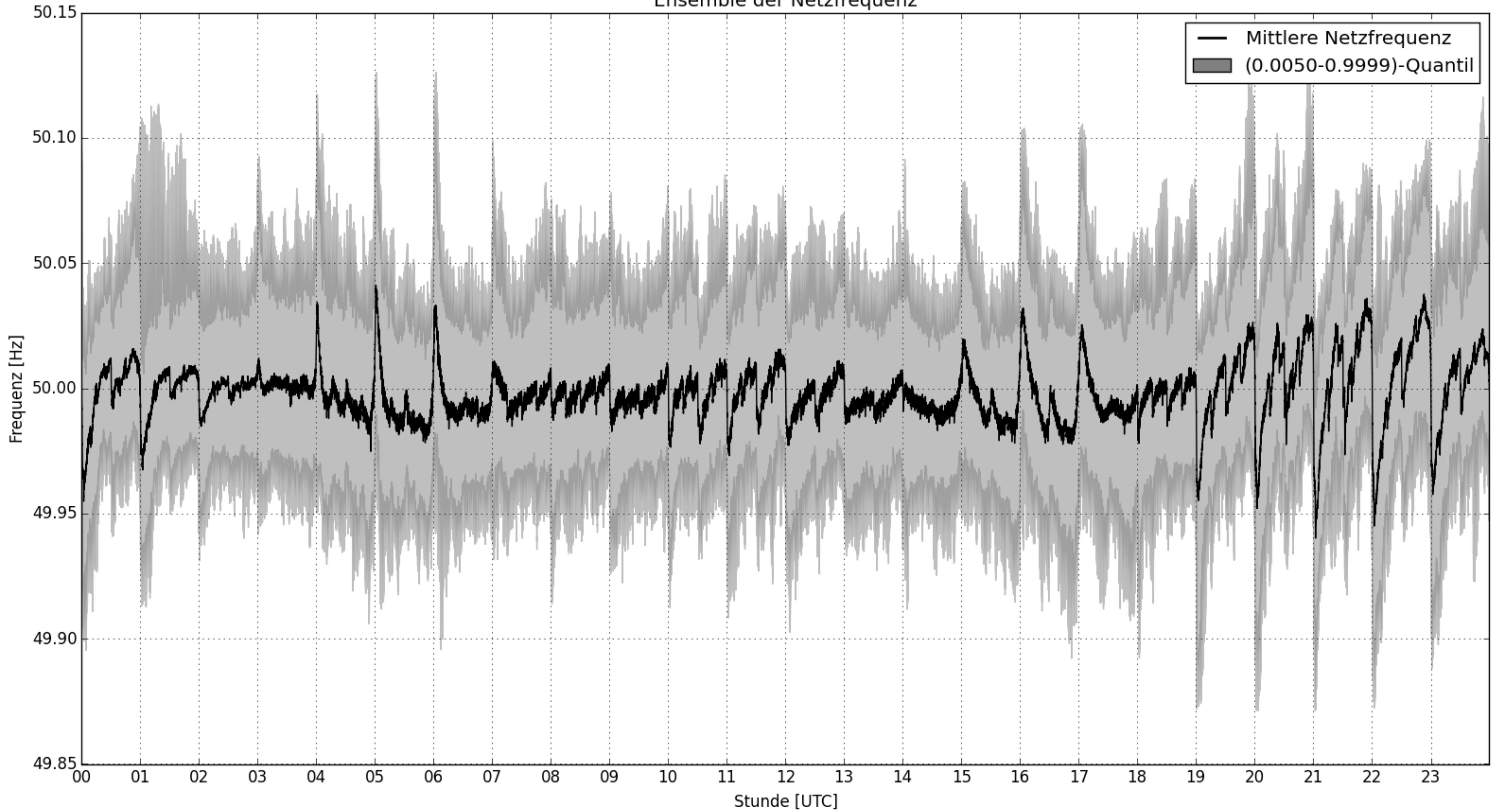
Ensemble der Netzfrequenz
